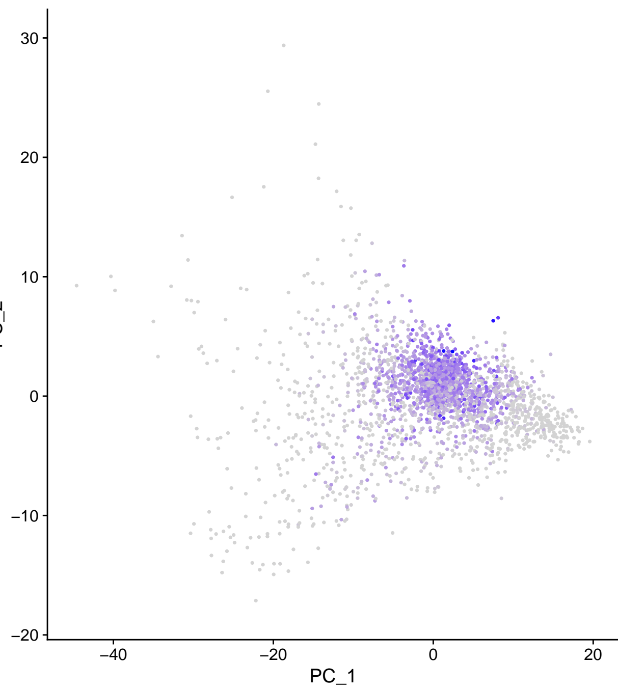
MALAT1
