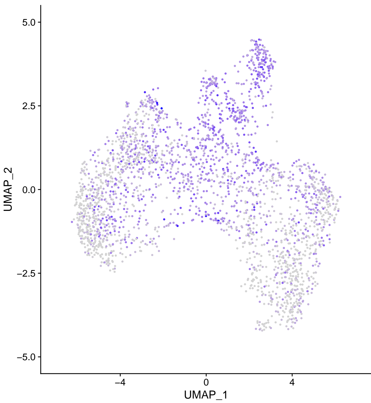
MALAT1
