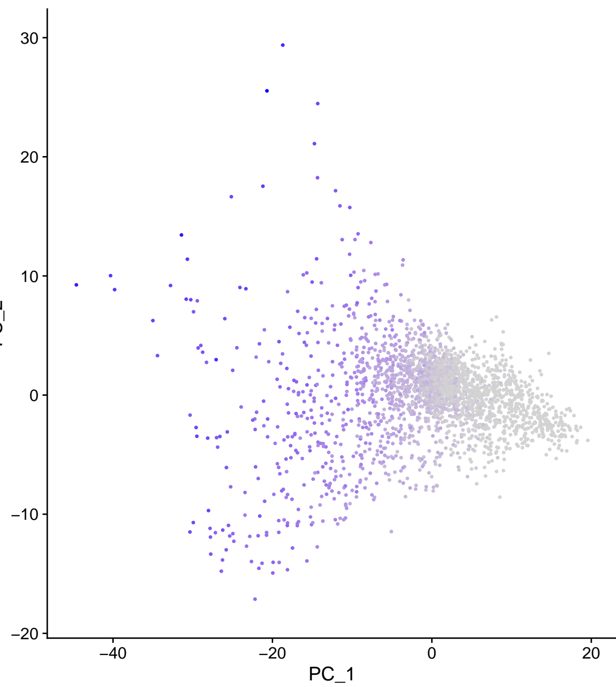
MALAT1
