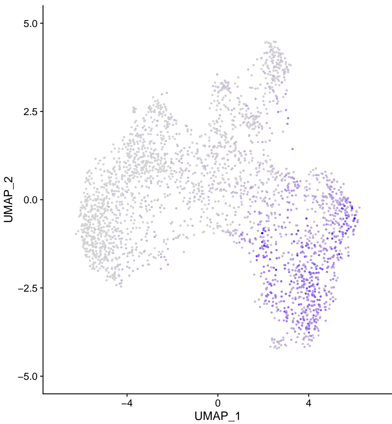
MALAT1
