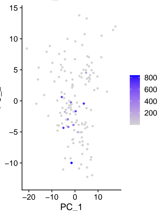
m_NBEAL1
