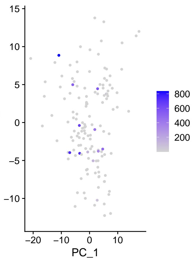
m_MAP2K7
