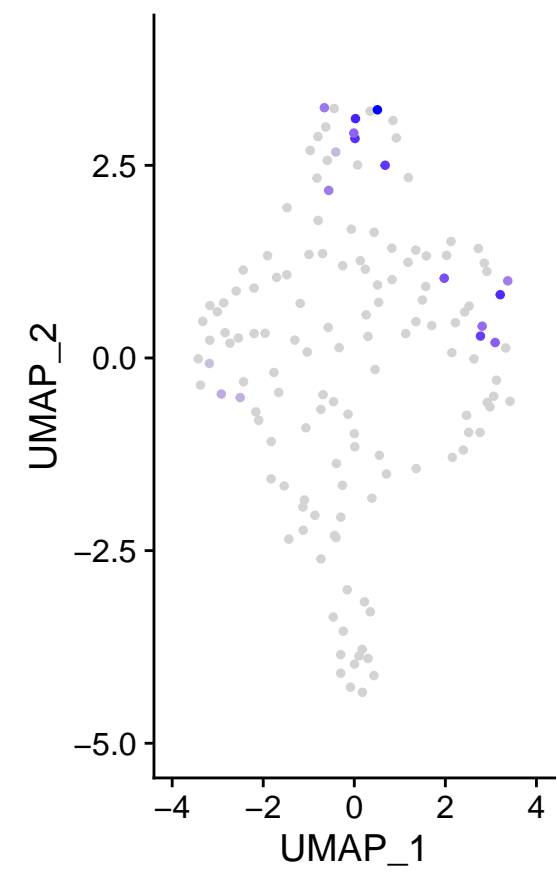
m_MAP2K7
