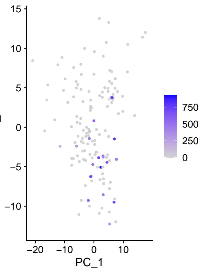
m_ID2
