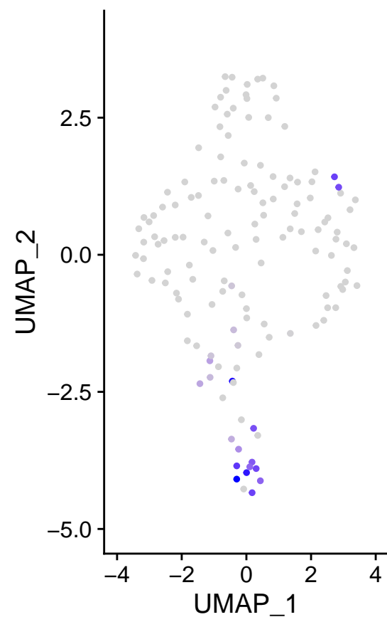
m_MAGED2
