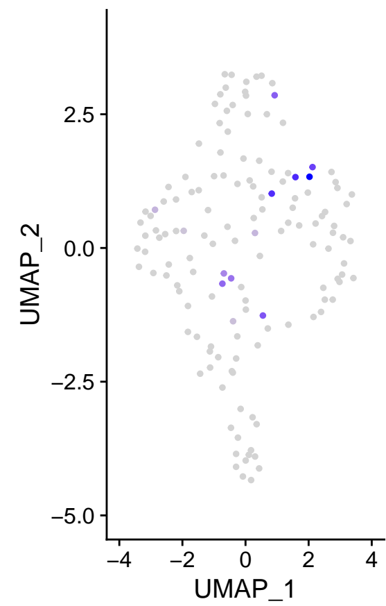
m_MAP2K7
