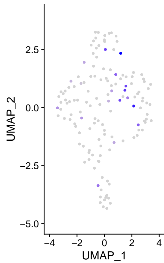
m_MAGED2
