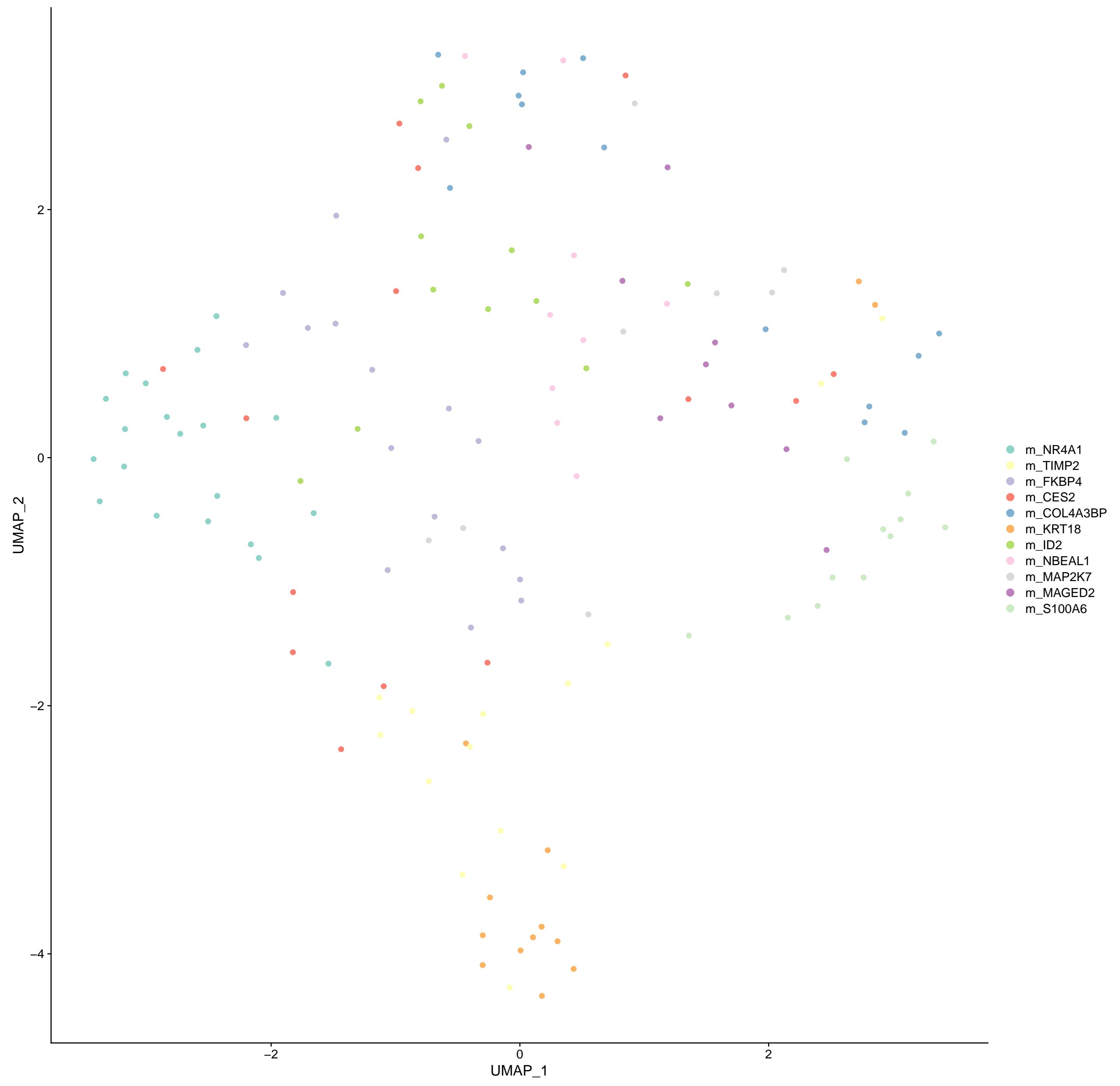
nmf
