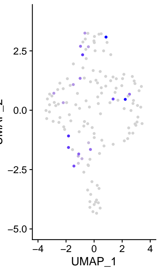
m_NBEAL1
