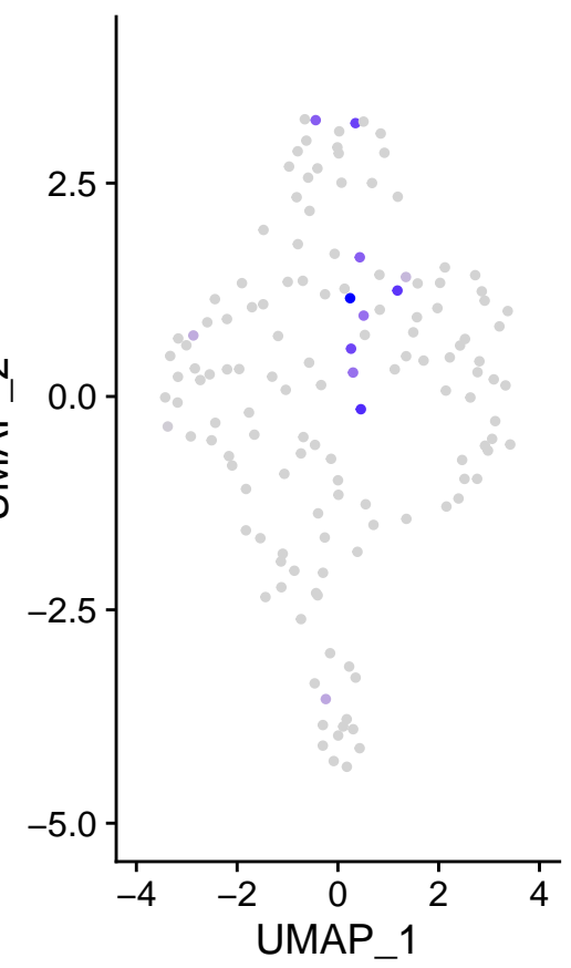
m_NBEAL1
