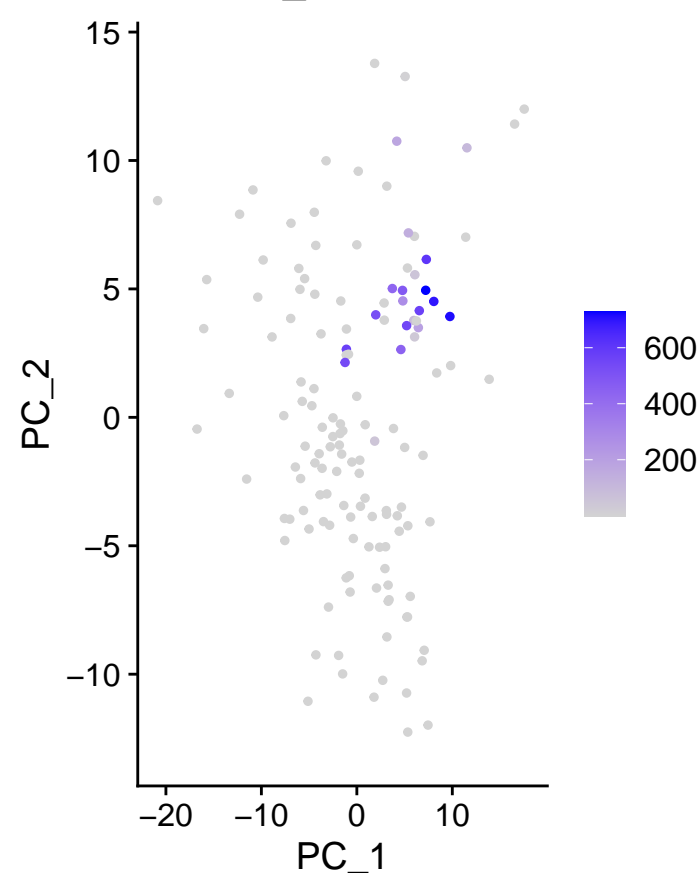
m_MAGED2
