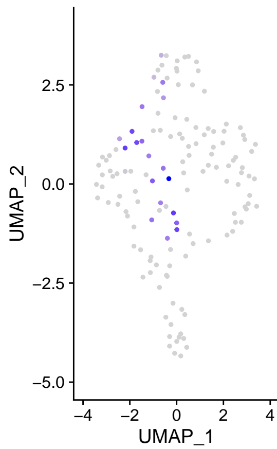
m_ID2
