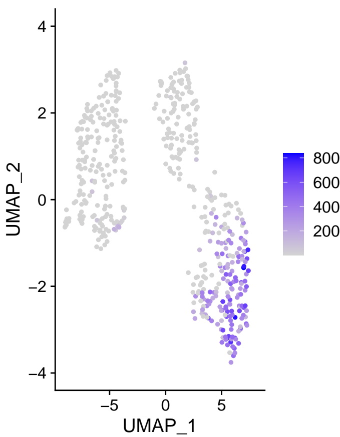
m_SPP1
