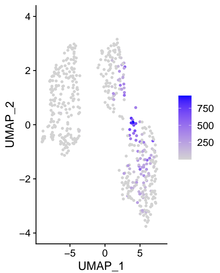
m_SRGN
