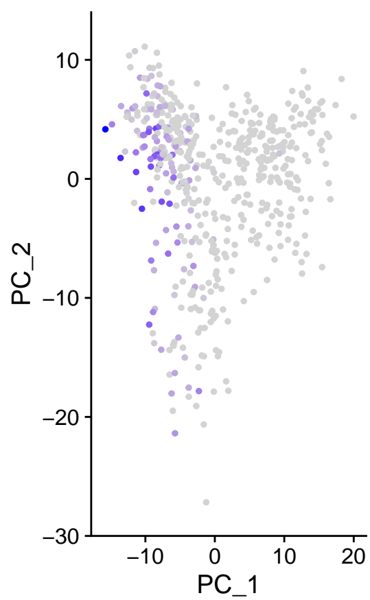
m_SRGN
