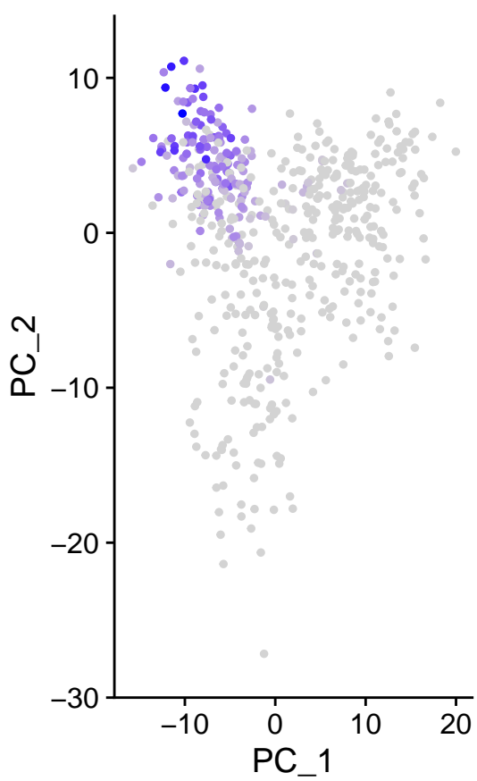
m_SPP1
