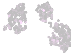
NPC
