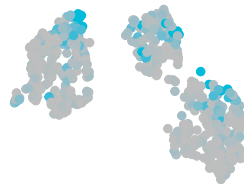
pEMT
