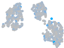
Alveolar
