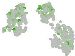
Oxphos
