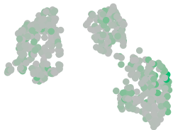
Metal
