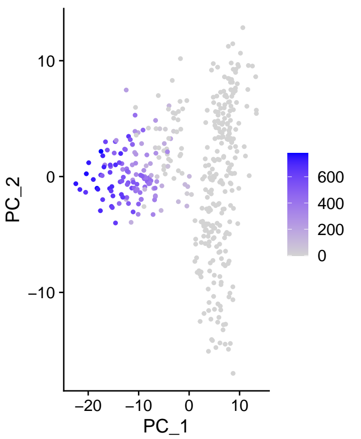
m_TPPP3
