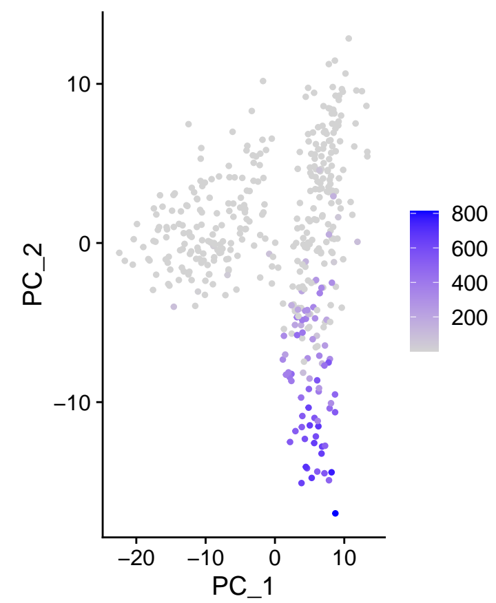
m_ADM
