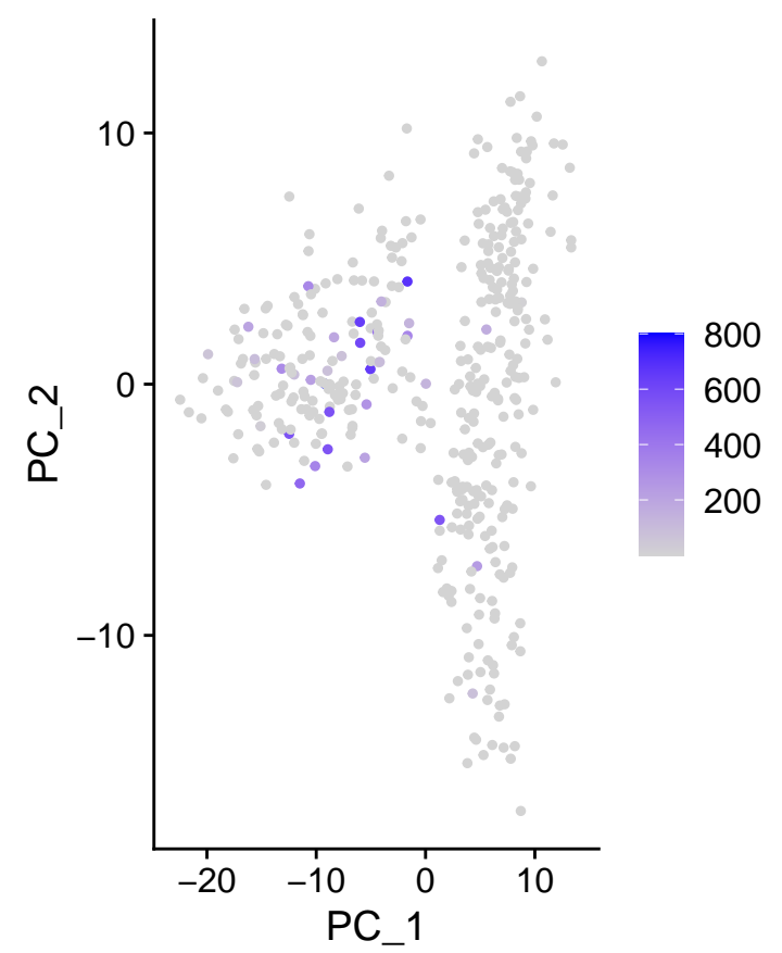
m_DCLRE1C
