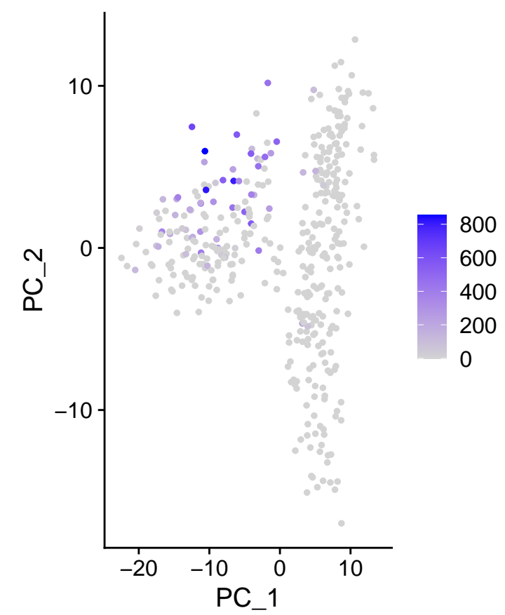
m_DNAAF1
