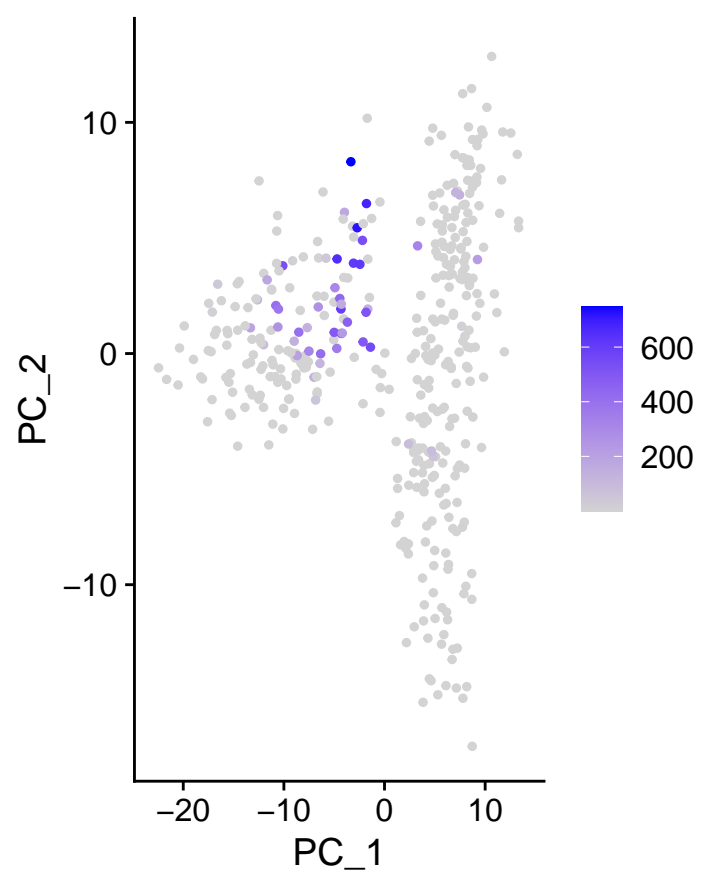
m_LAMB3
