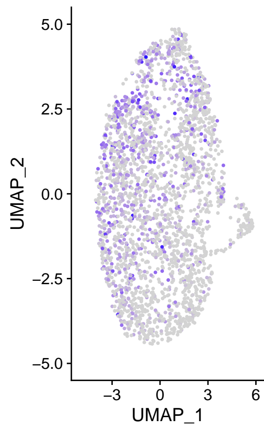
m_FAAP100
