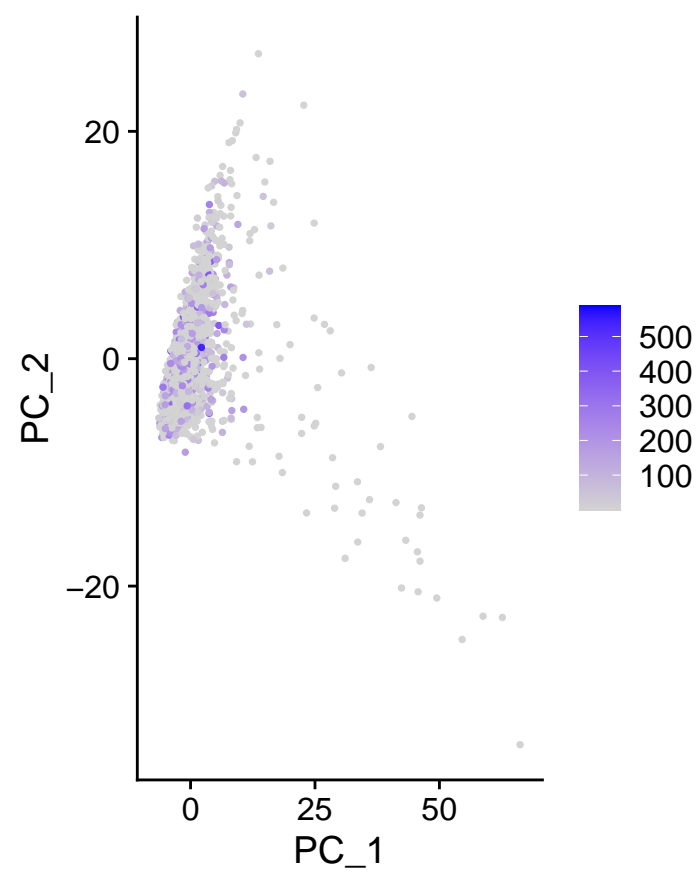
m_IGKC
