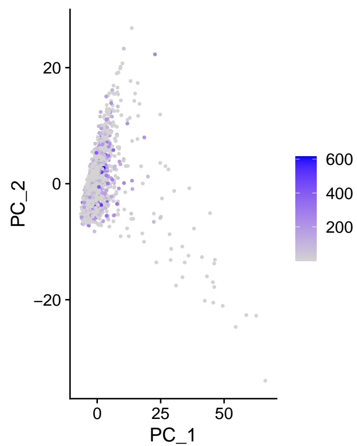
m_IGKC
