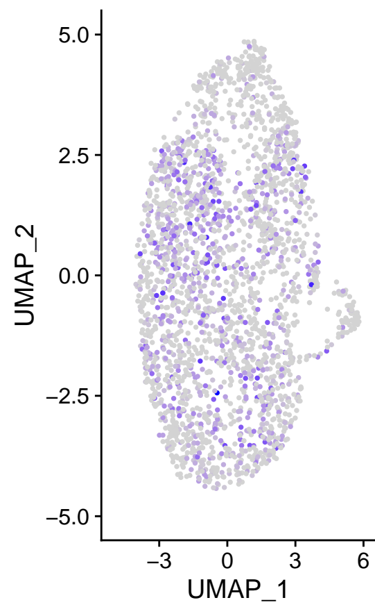
m_IGKC
