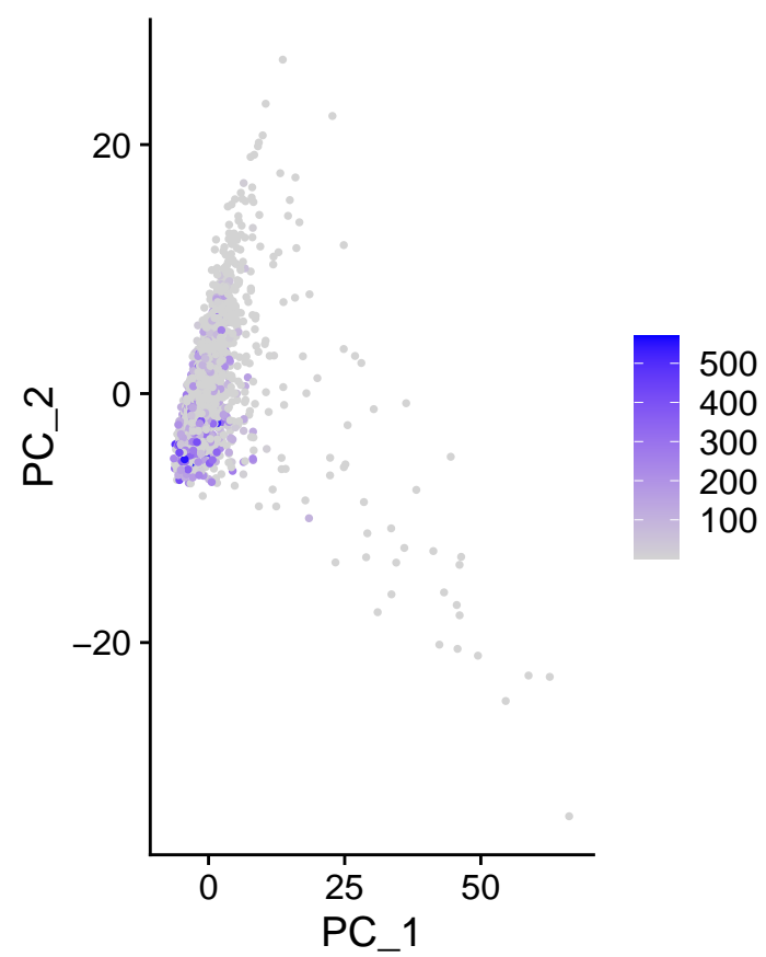
m_FAAP100
