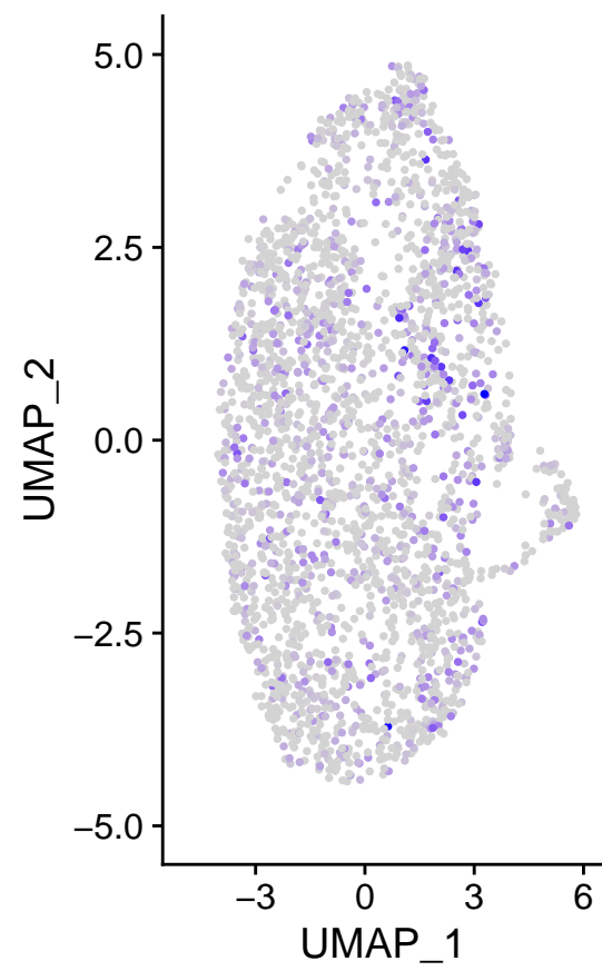
m_IGKC
