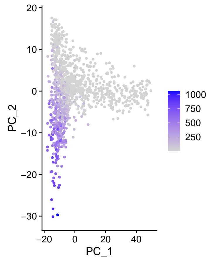
m_FAM50A
