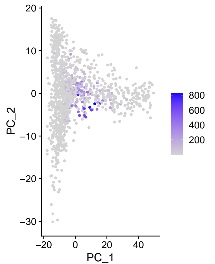
m_GPX3
