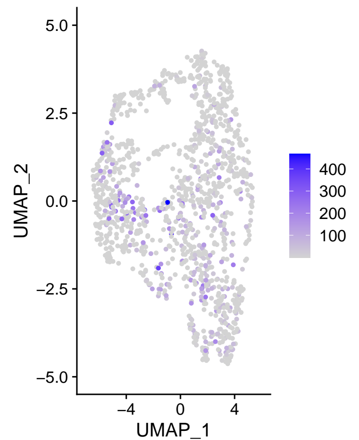
m_FAM50A
