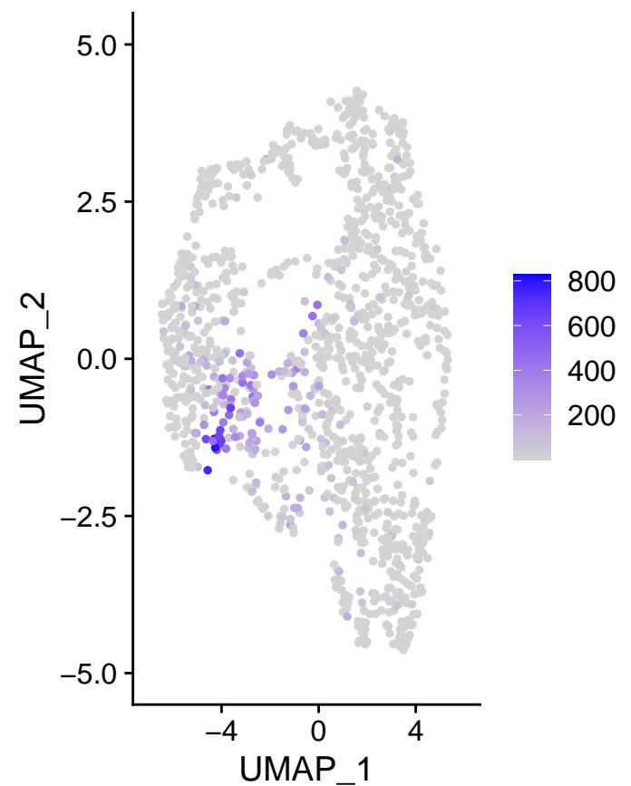
m_GPX3
