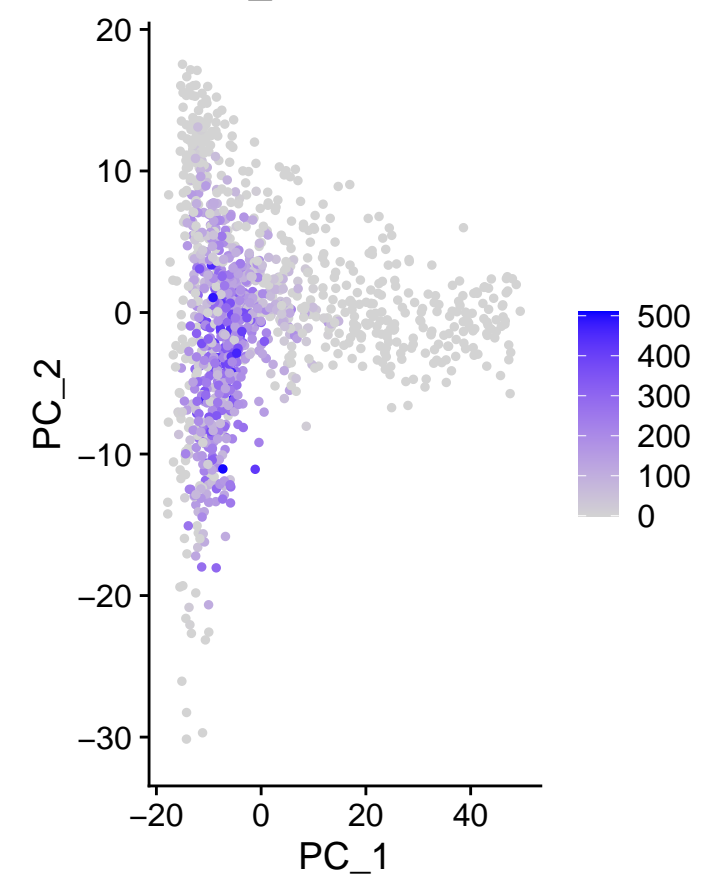
m_IGKC
