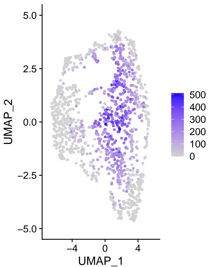
m_IGKC
