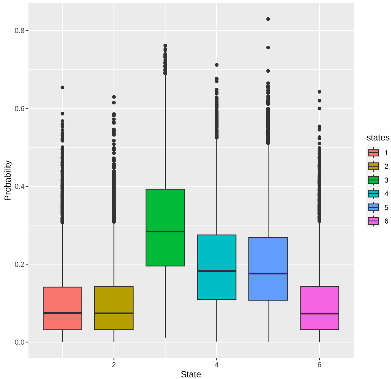
chr5-region_1145
