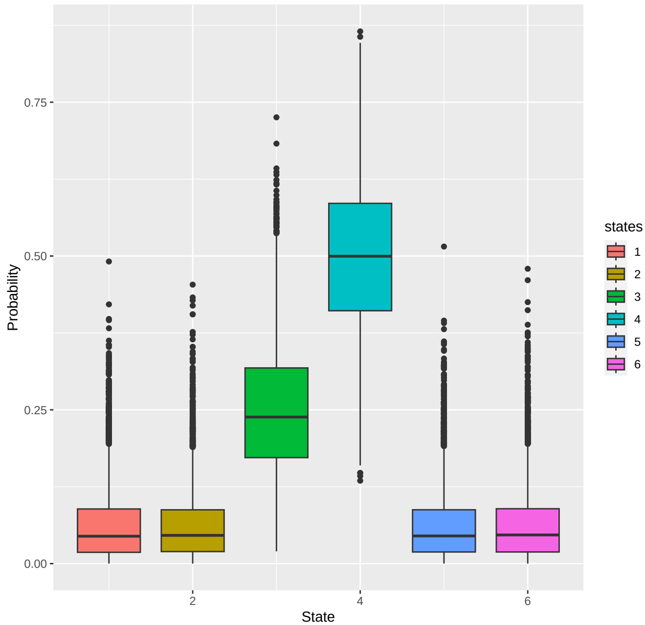
chr9-region_3535
