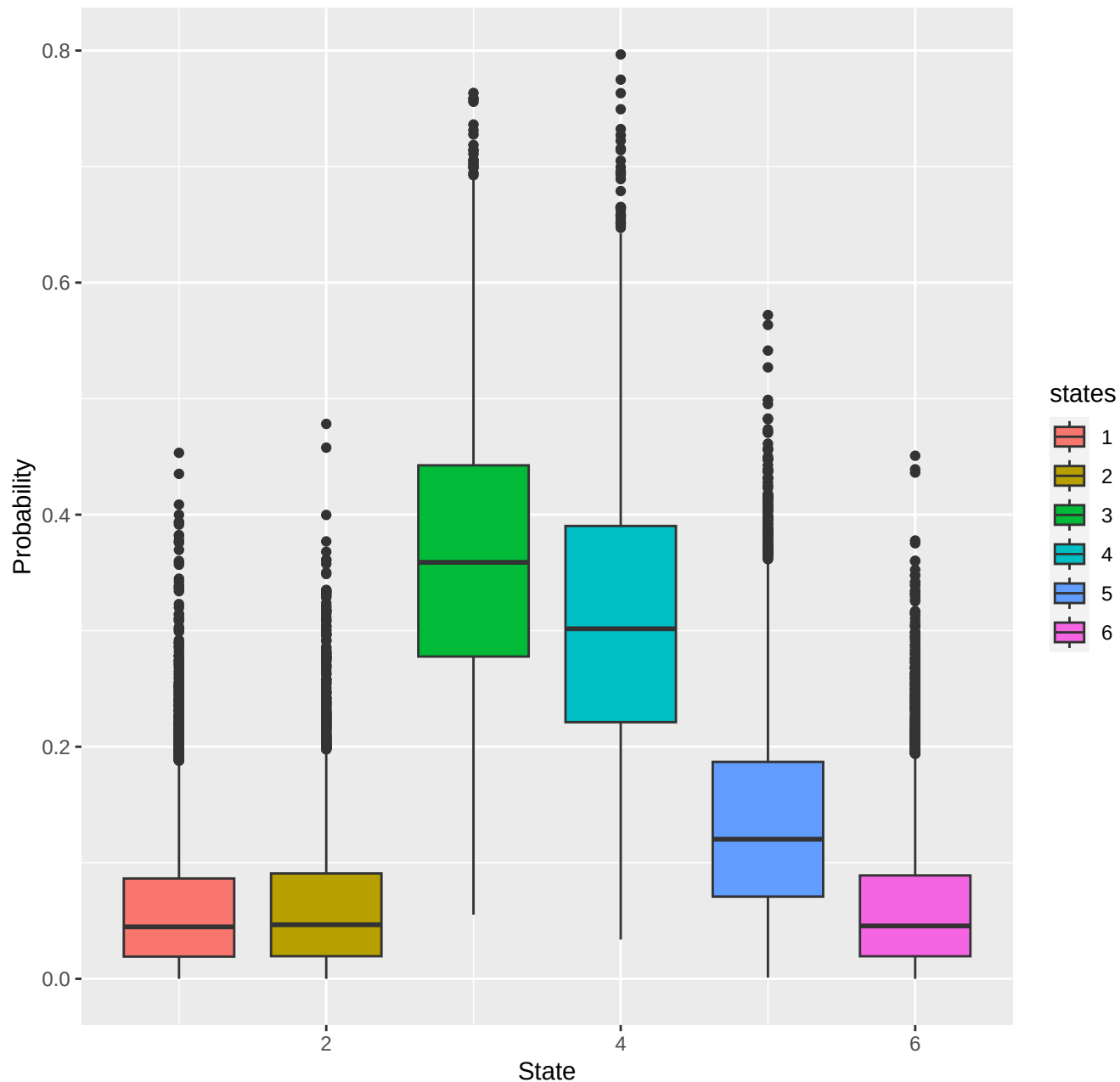
chr5-region_619
