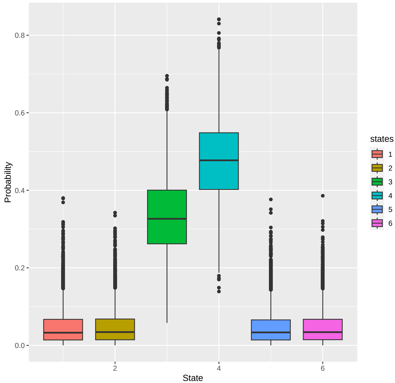
chr16-region_85
