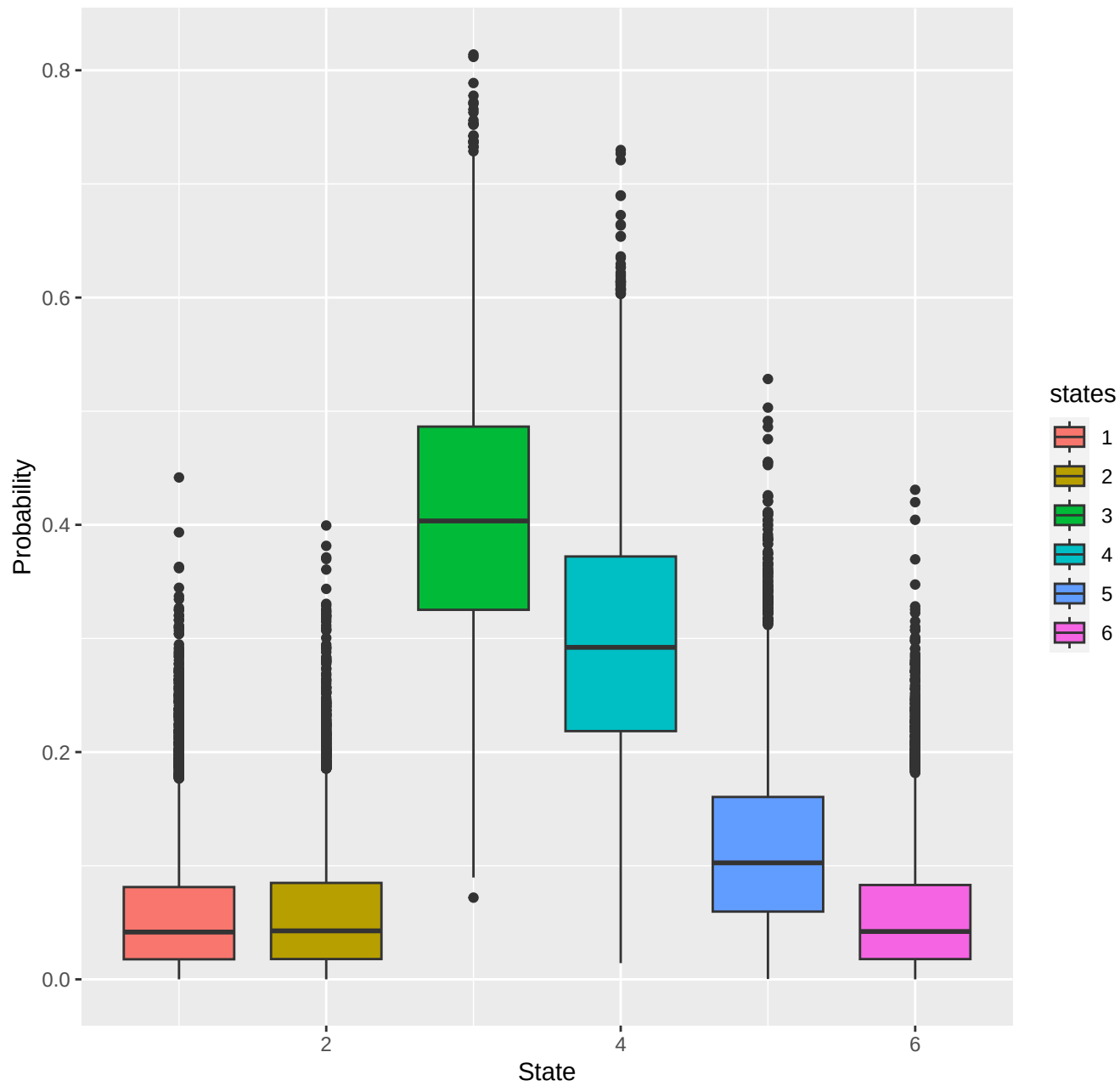
chr15-region_2164
