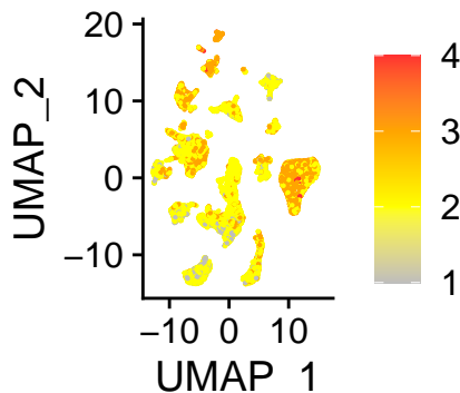
Oxphos1
