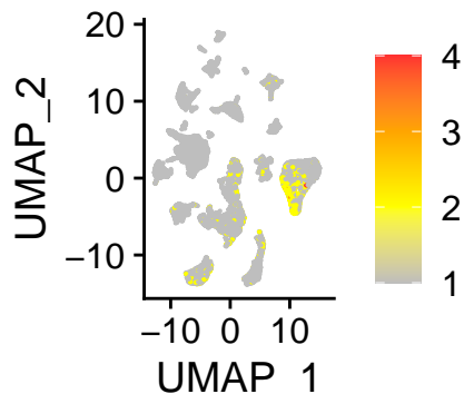
NPC_like1
