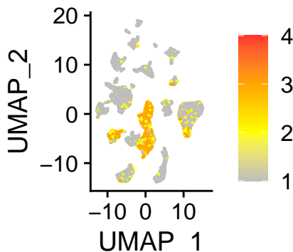
OPC_like_UCell
