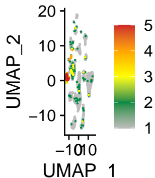
T.cells7
