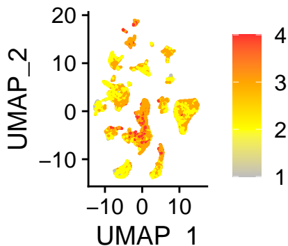
pEMT_UCell
