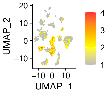
OPC_like1
