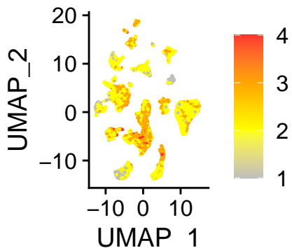
pEMT1
